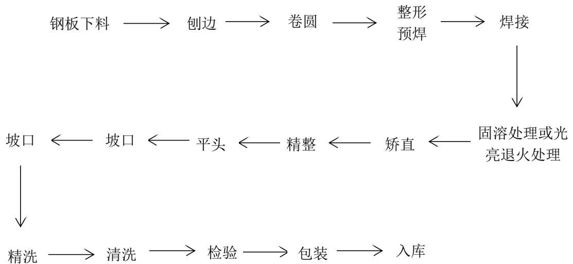
图 2.2-1 高性能大口径不锈钢焊管工艺流程图
