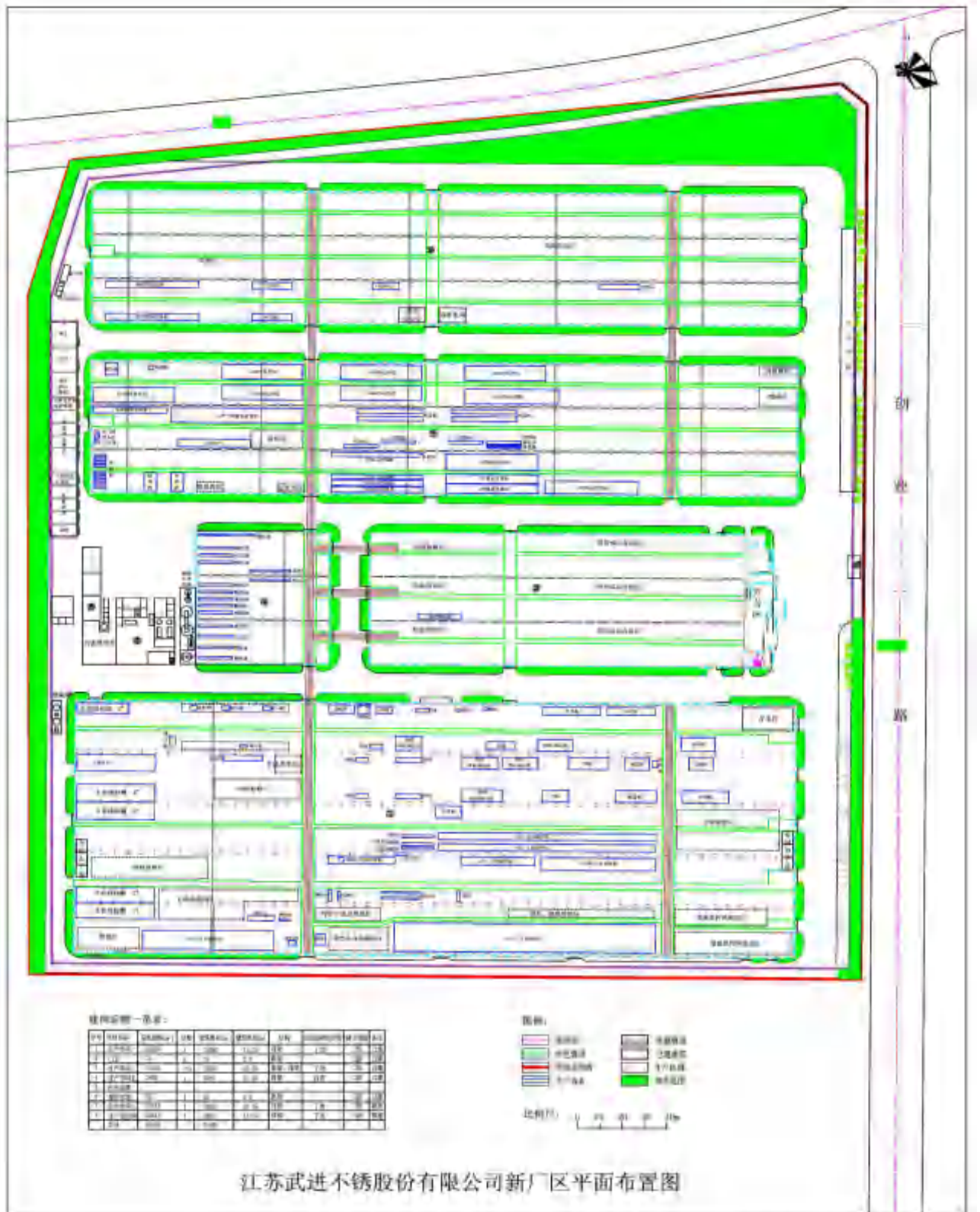
图1.2-2 厂区平面布置图
