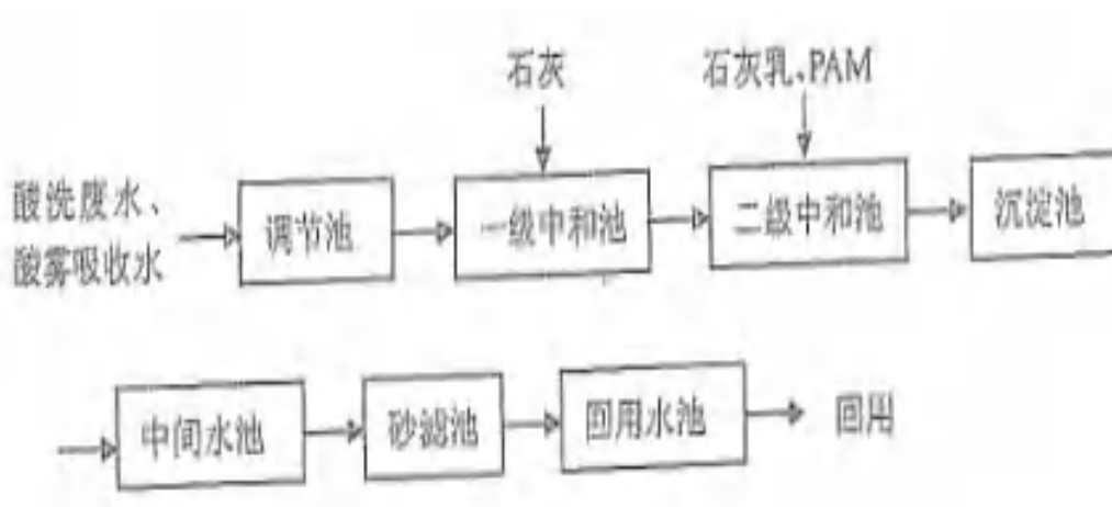
图 2.3-1 废水处理流程图
